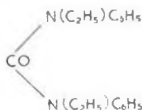
Fig. 29 Carbamite
