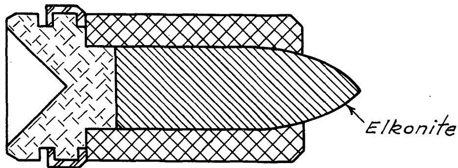
Fig. 5. Solid sabot CW1e.
