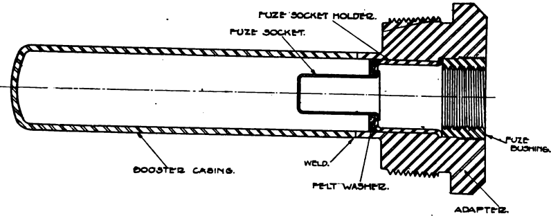
ADAPTER & BOOSTER MARK VI.
