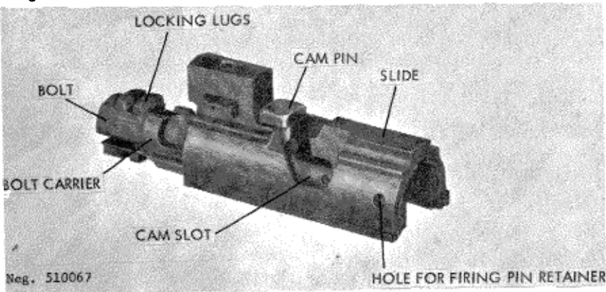
Figure 68. C.A.L. bolt.
