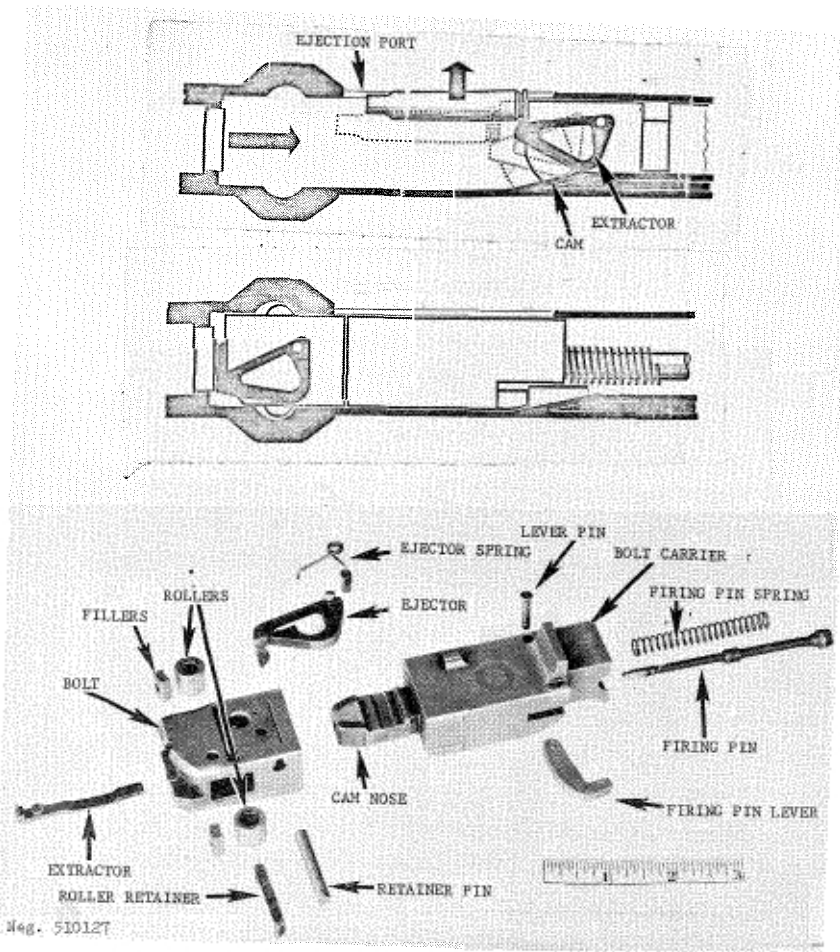
Figure 128. StG 57 bolt.
